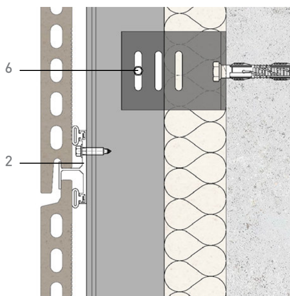
C. Placement in vertical profile Colocación en perfil vertical
