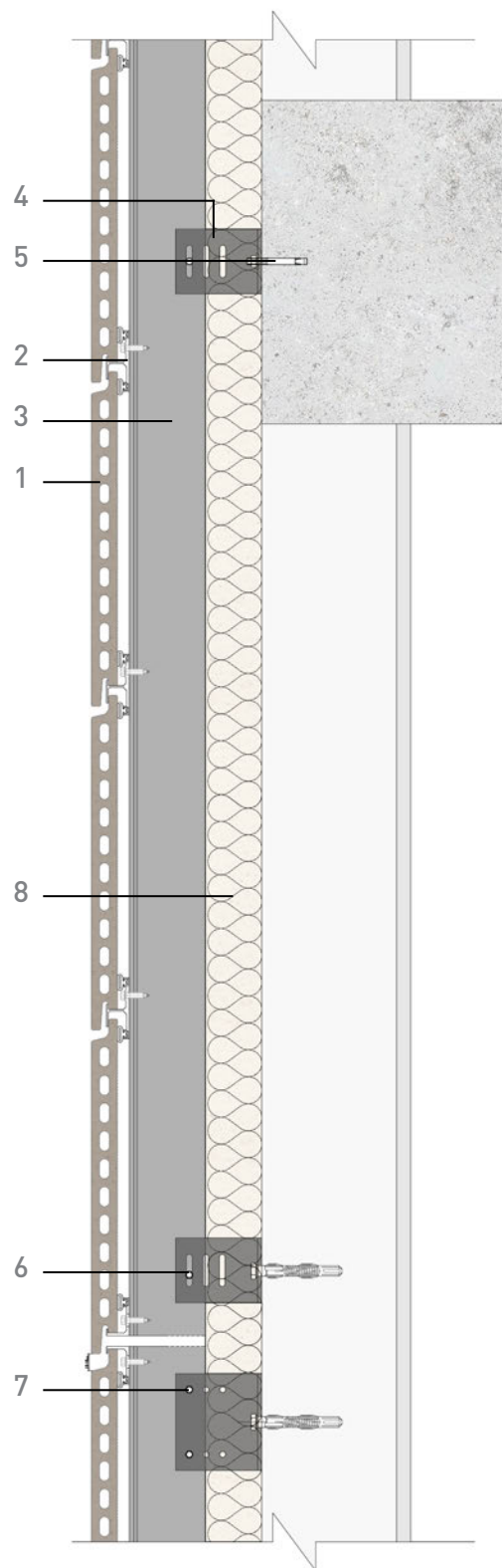
A. Vertical section Sección vertical
