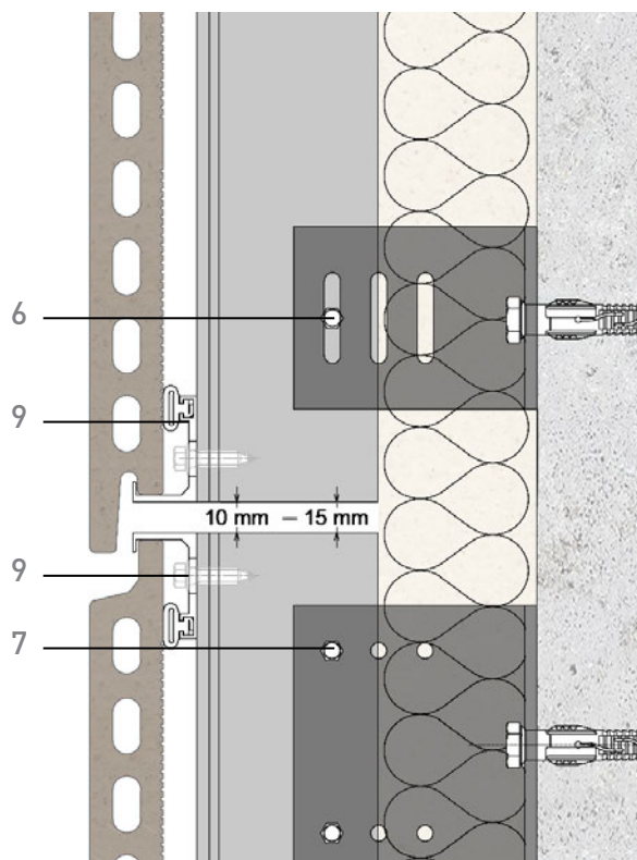
B. Detail of mounting fixings Detalle de montaje de fijaciones
